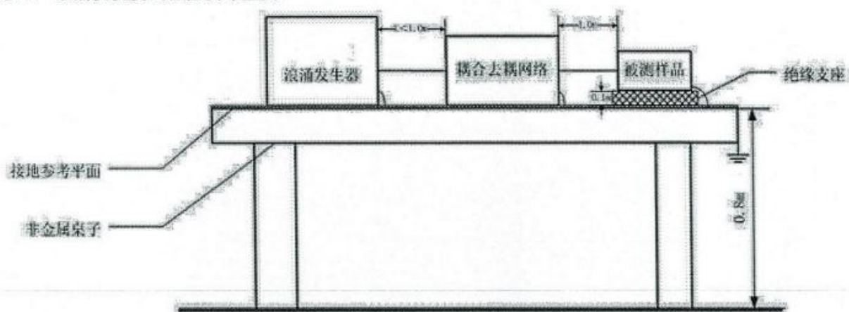
图 9 浪涌抗扰度试验检测布置图
