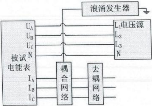
图 14 浪涌抗扰度试验接线图(电流线路)
