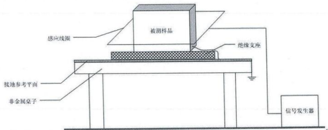
附录 3 工频磁场抗扰度试验接线布置图
