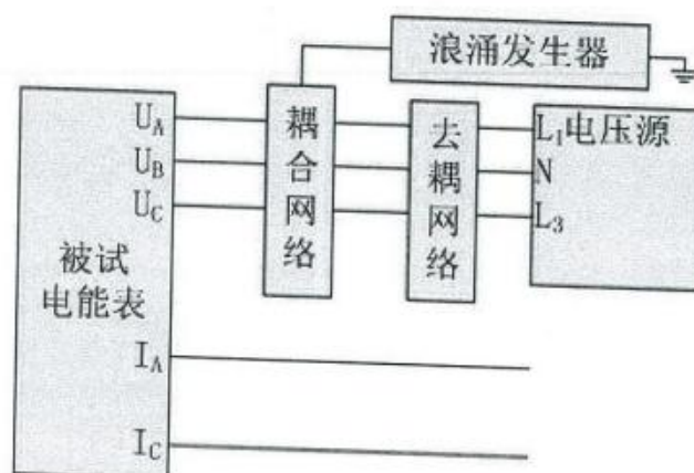
图 15 浪涌抗扰度试验接线图(电压线路)
