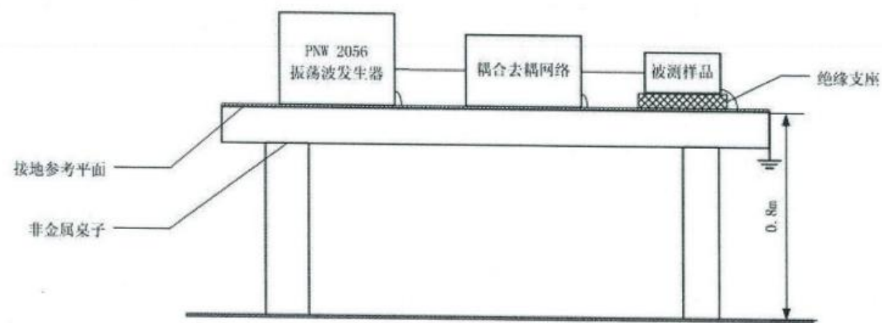
图 11 衰减振荡波抗扰度试验布置图
