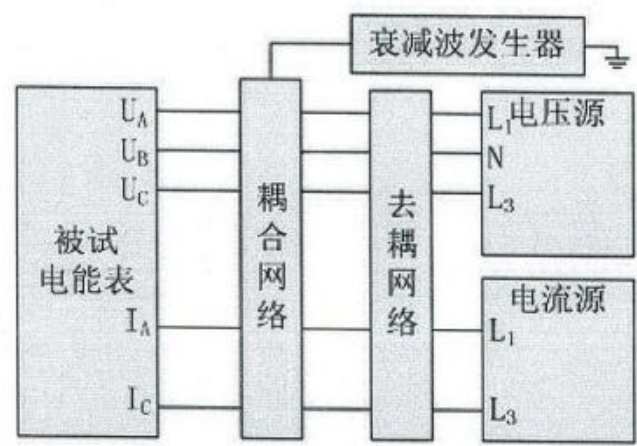
图 12 衰减振荡波抗扰度试验接线图
