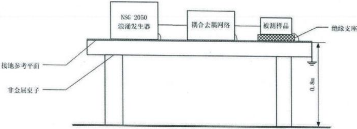
图 13 浪涌抗扰度试验布置图
