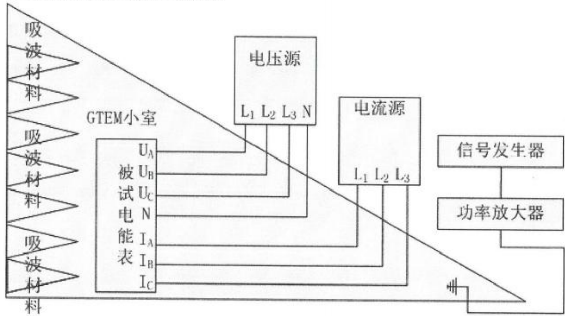
图 7 射频电磁场抗扰度试验接线布置图
