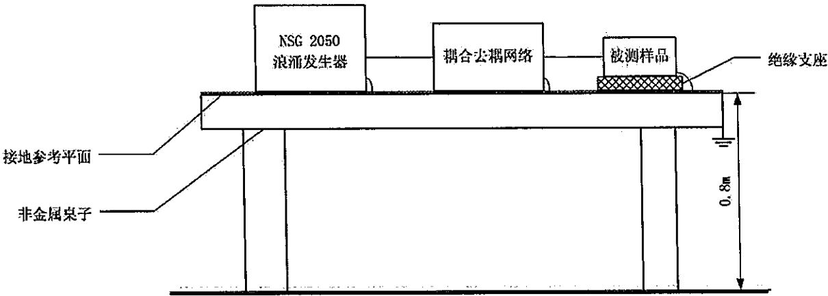
附录 10 浪涌抗扰度试验布置图
