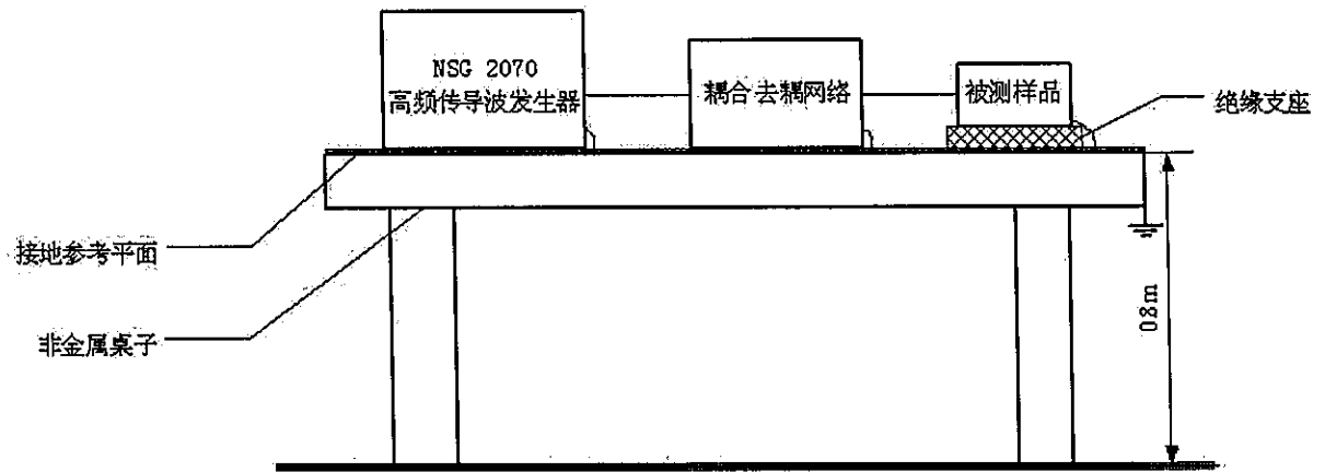
图 4 射频场感应的传导骚扰抗扰度试验布置图
