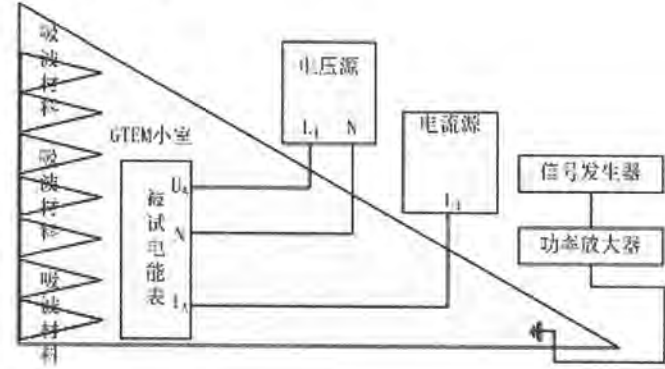
附录 7 射频电磁场试验接线布置图
