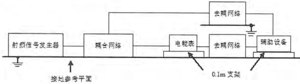
附录 4 射频场感应的传导干扰试验布置图
