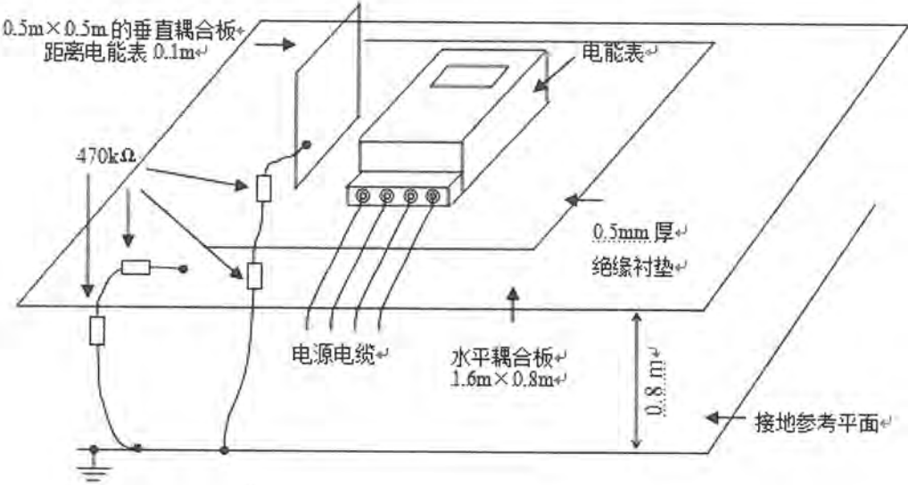
附录 6 静电放电试验接线布置图
