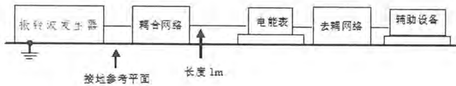
图 15 振铃波试验布置图
