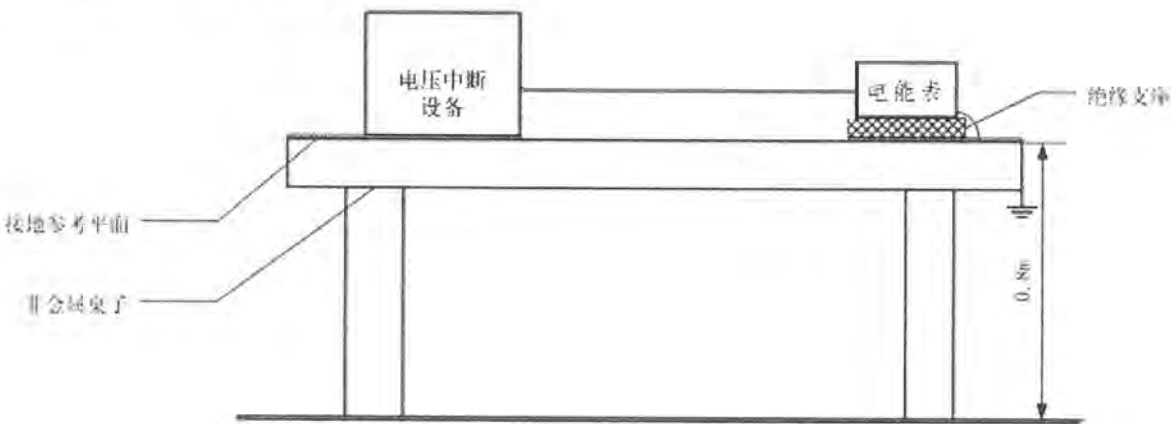
附录 1 电压暂降和短时中断试验布置图
