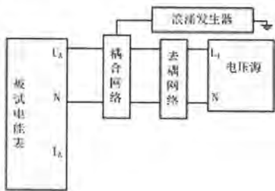
附录 12 浪涌试验接线图（电网电源端口）
