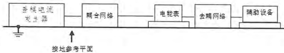
附录 14 传导差模电流干扰试验布置图
