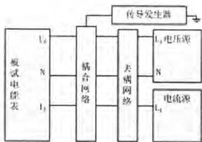
附录 5 射频场感应的传导干扰试验接线图
