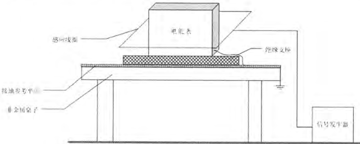
附录 3 外部工频磁场试验接线布置图
