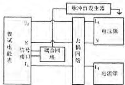
附录 10 快速瞬变脉冲群试验接线图（信号端口）
