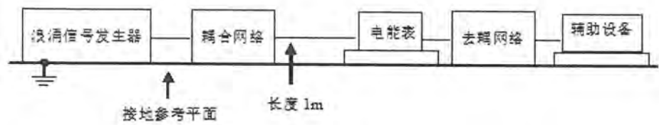
附录 11 浪涌试验布置图
