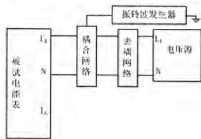
附录 16 振铃波试验接线图（电网电源端口）
