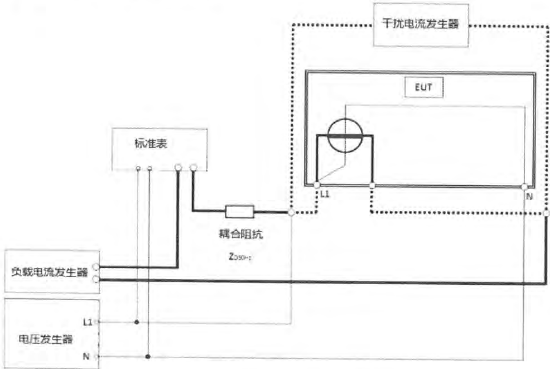
图 18 传导差模电流干扰试验接线图 以下空白
