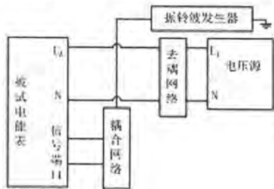
图 17 振铃波试验接线图（信号端口）
