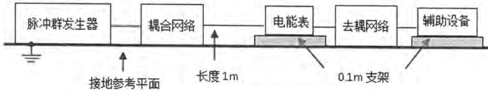
图 8 快速瞬变脉冲群试验布置图
